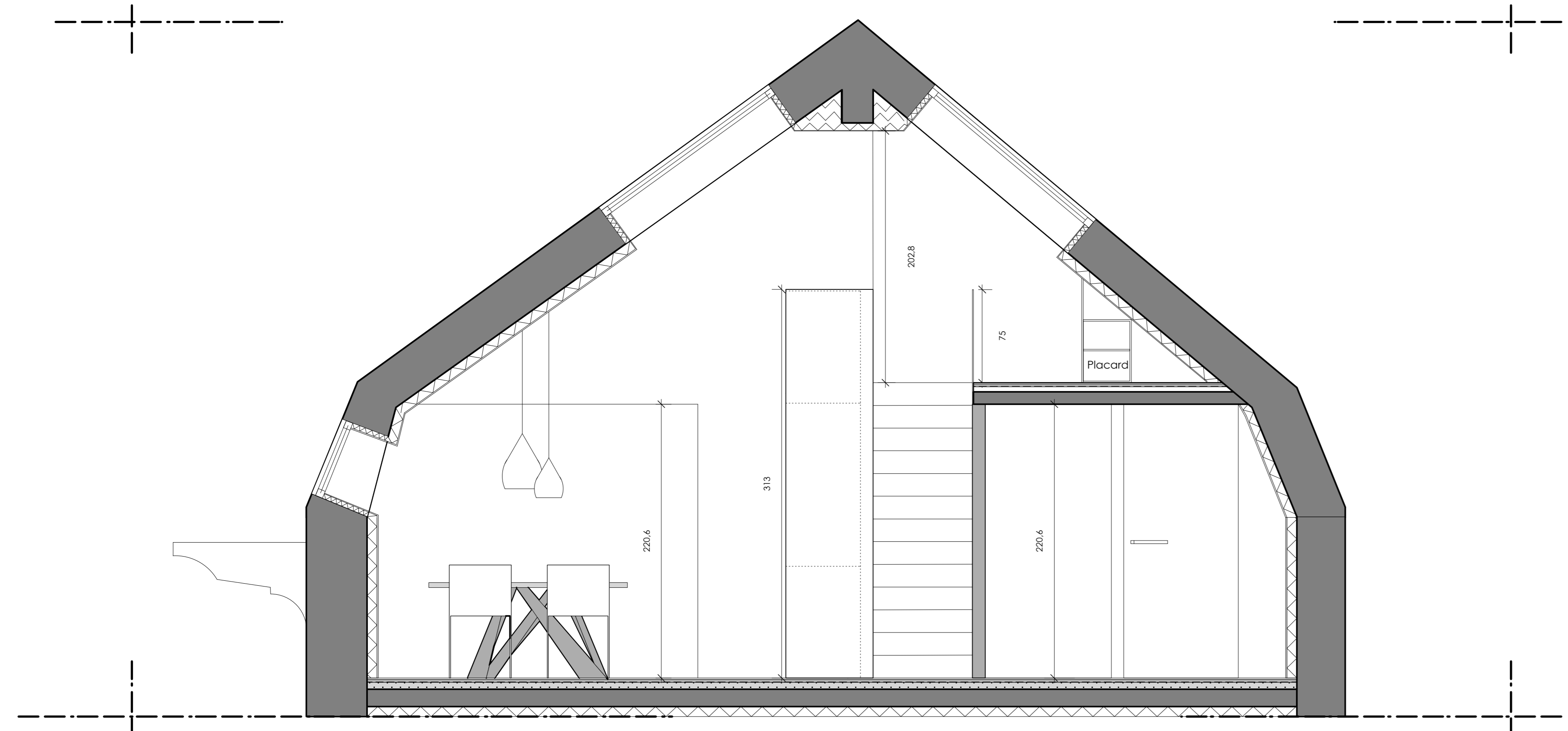
Coupe CC - studio 1/25
