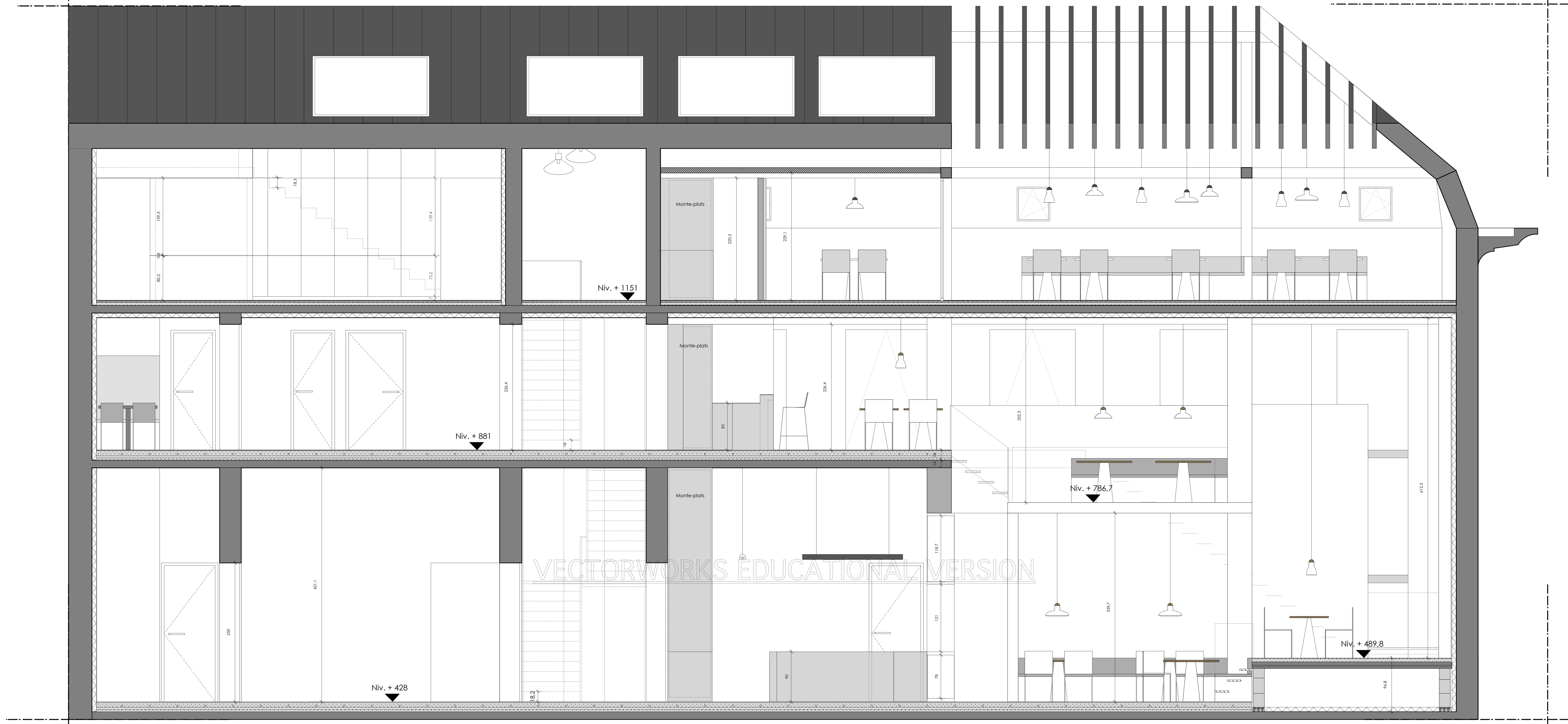
Coupe longitudinale AA 1/25
