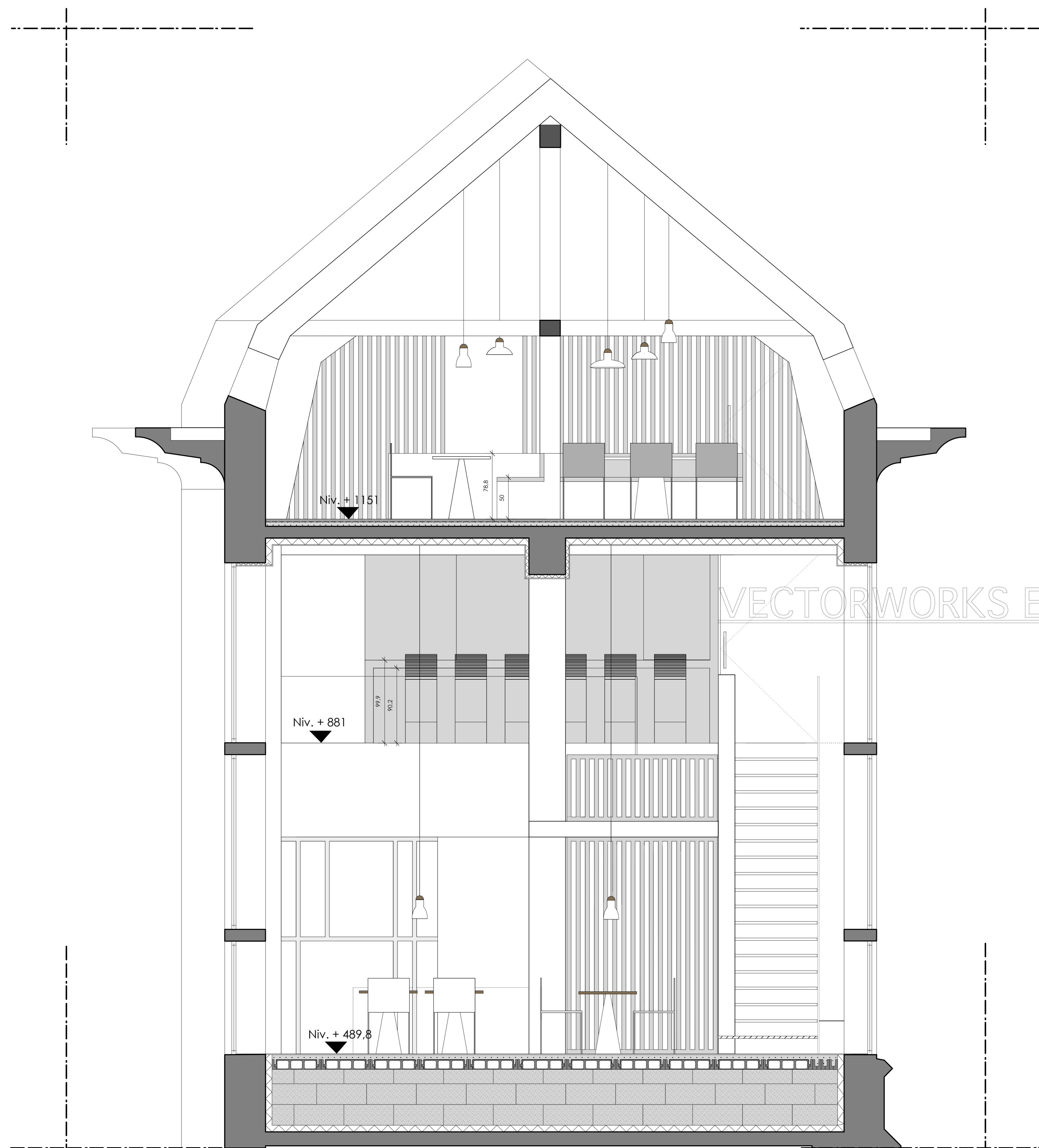
Coupe latérale BB 1/25
