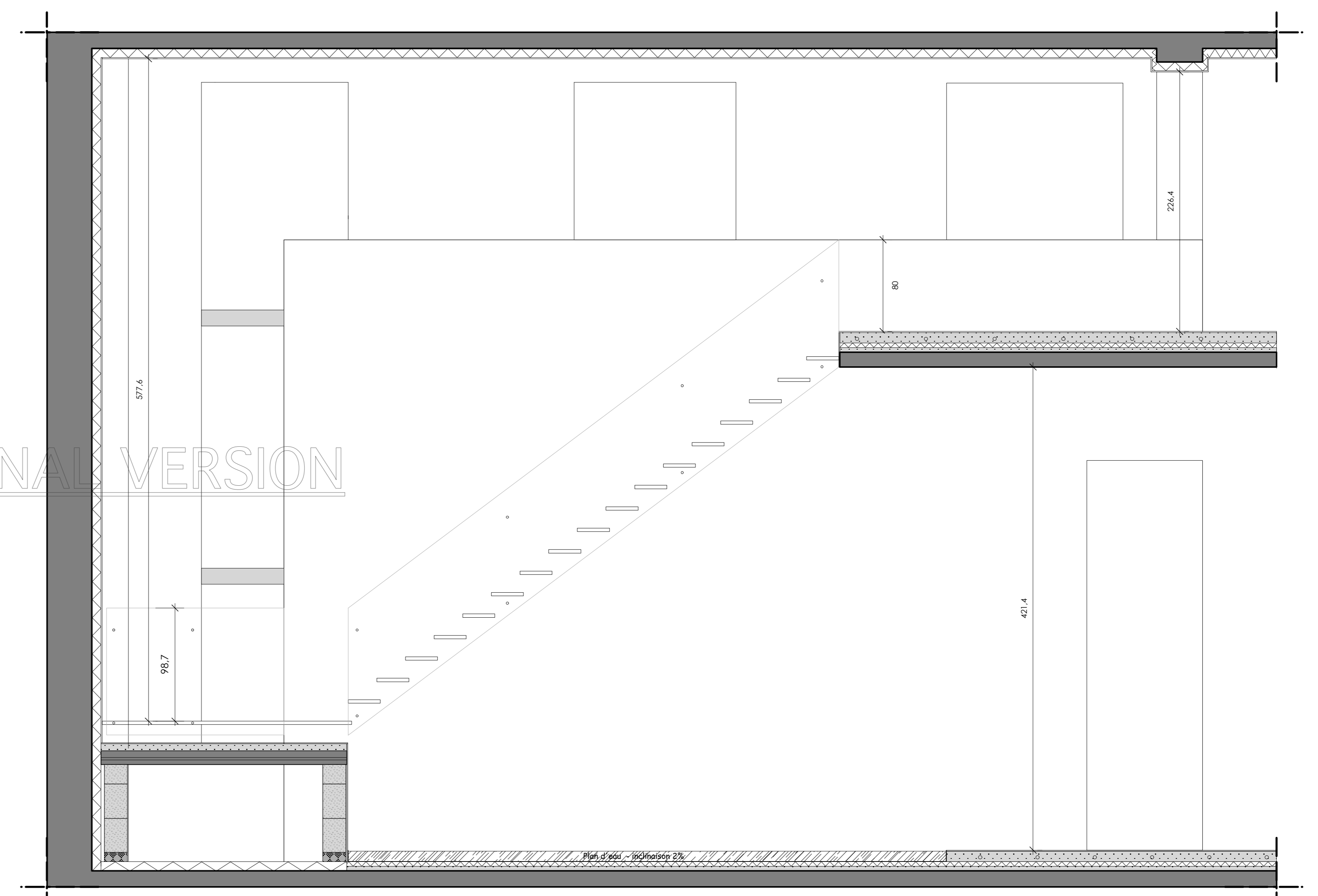
Section escalier restaurant 1/25
