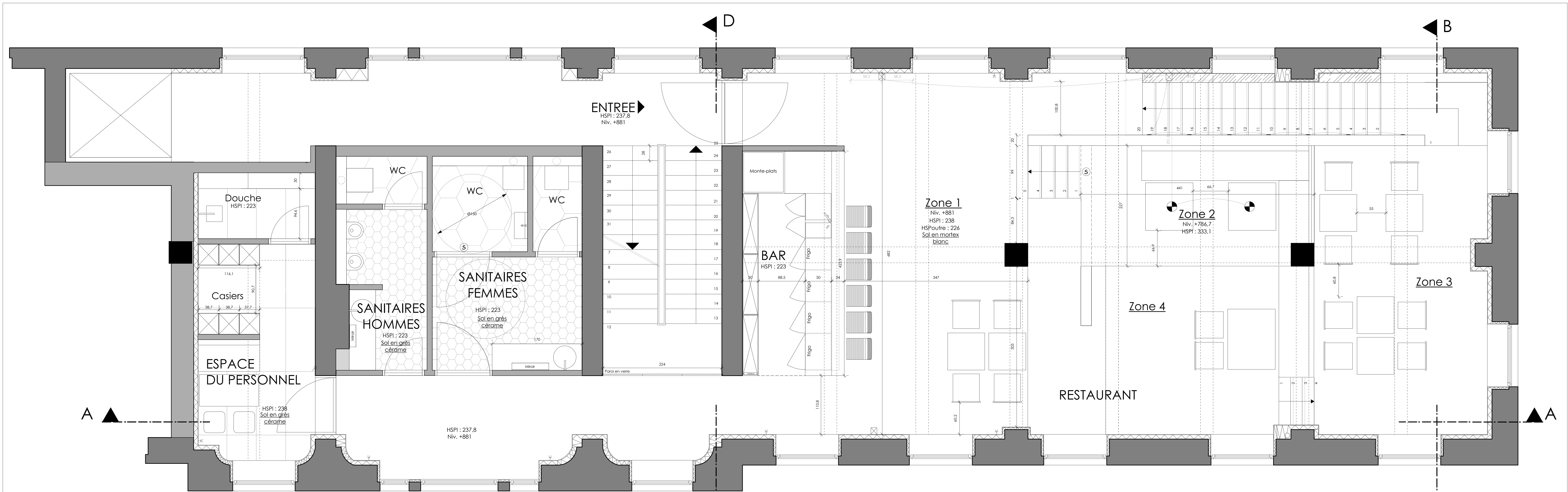
2ème étage 1/25
