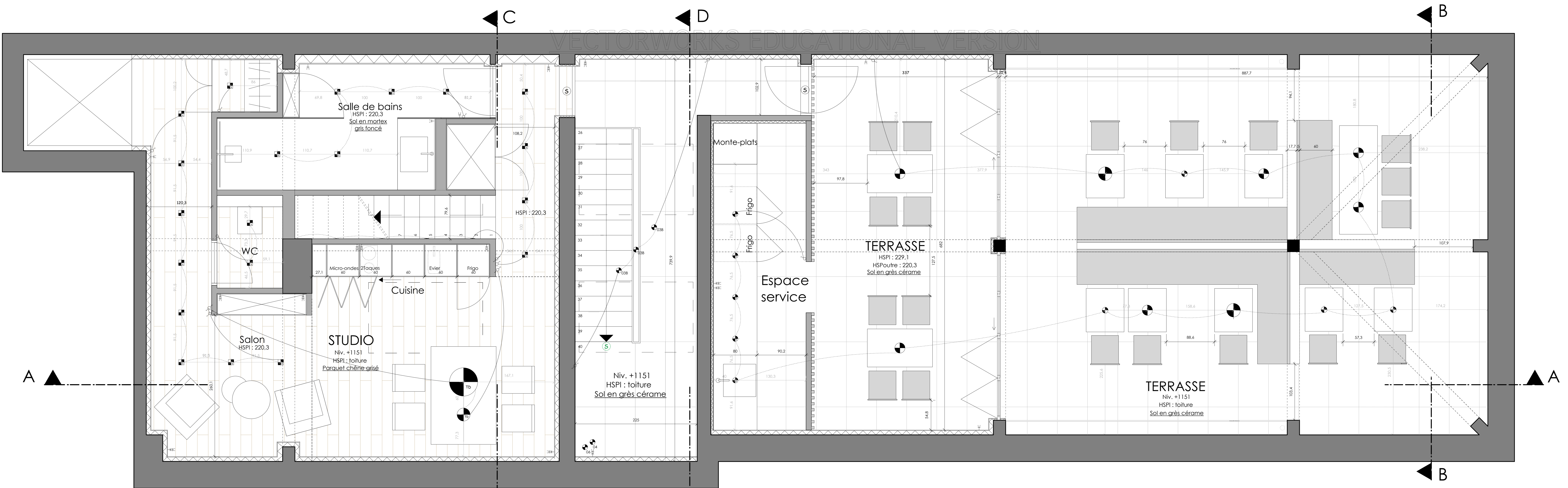
Combles 1/25
