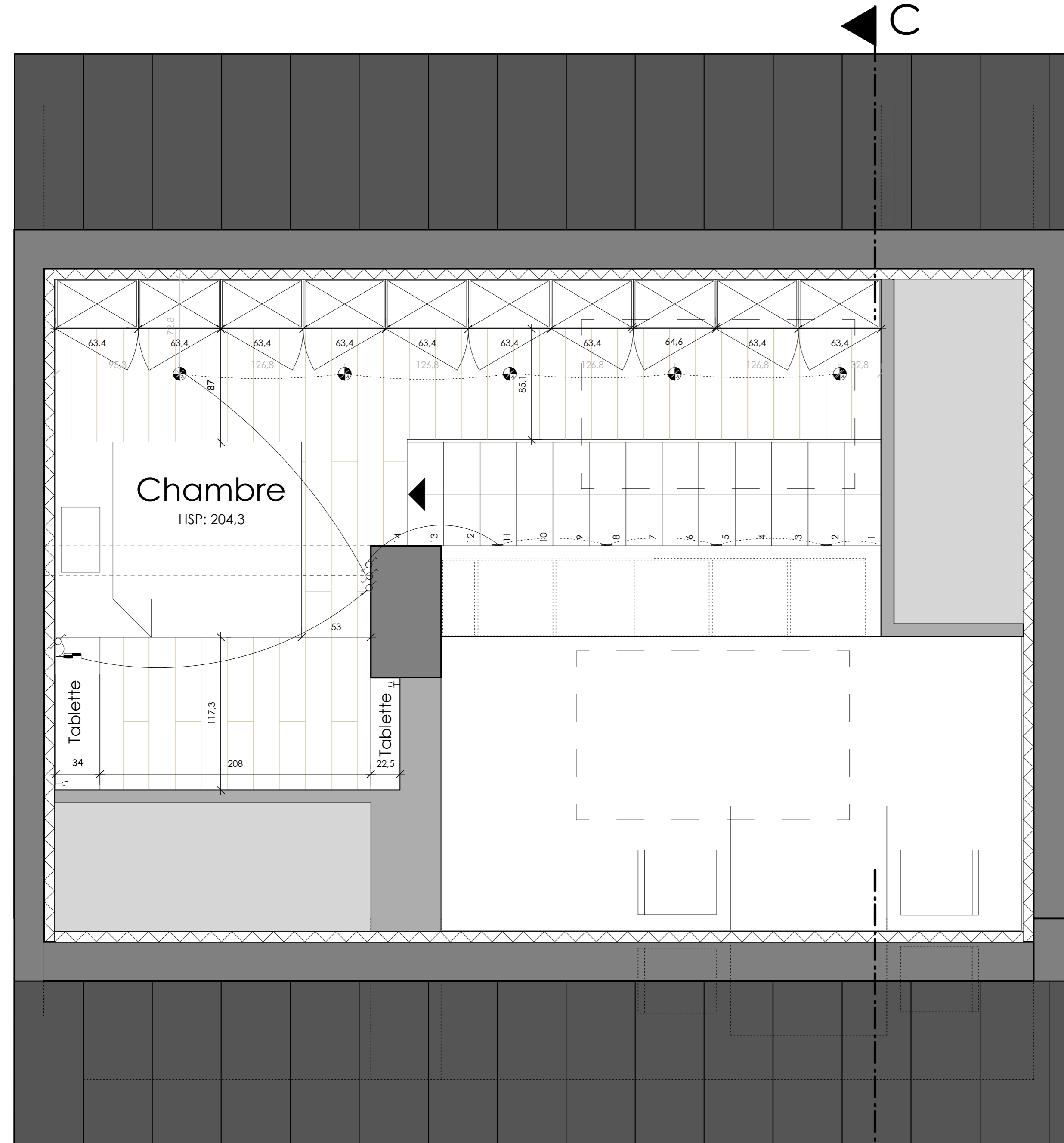
Combles 1/25
